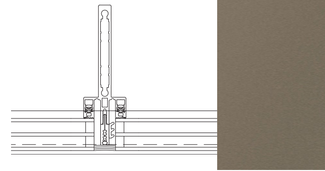
Pfosten Riegel Fassade | FWS 50 SG SI Schüco Innen und Außen: Eloxal A6/C33 Bronze
