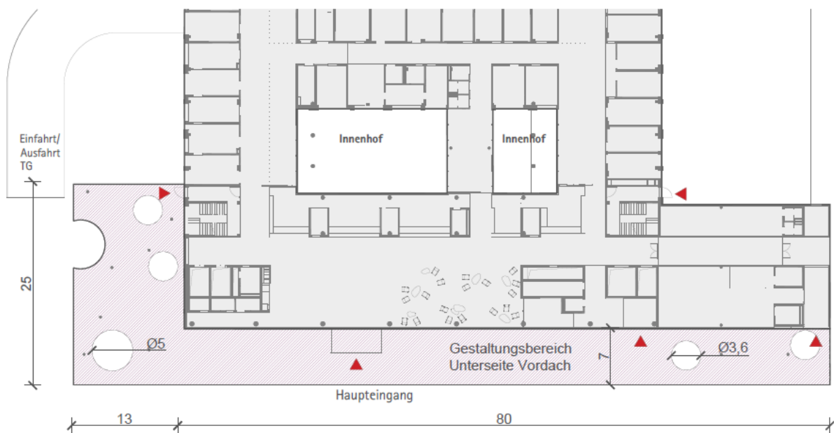
Abb 2. Grundriss
